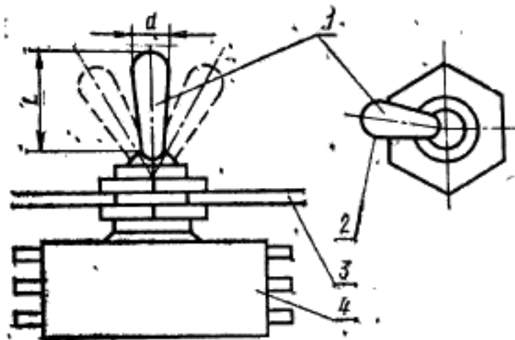
1 — приводной элемент; 2 — рабочая поверхность; 3 — панель; 4 — тумблер Черт. 1
