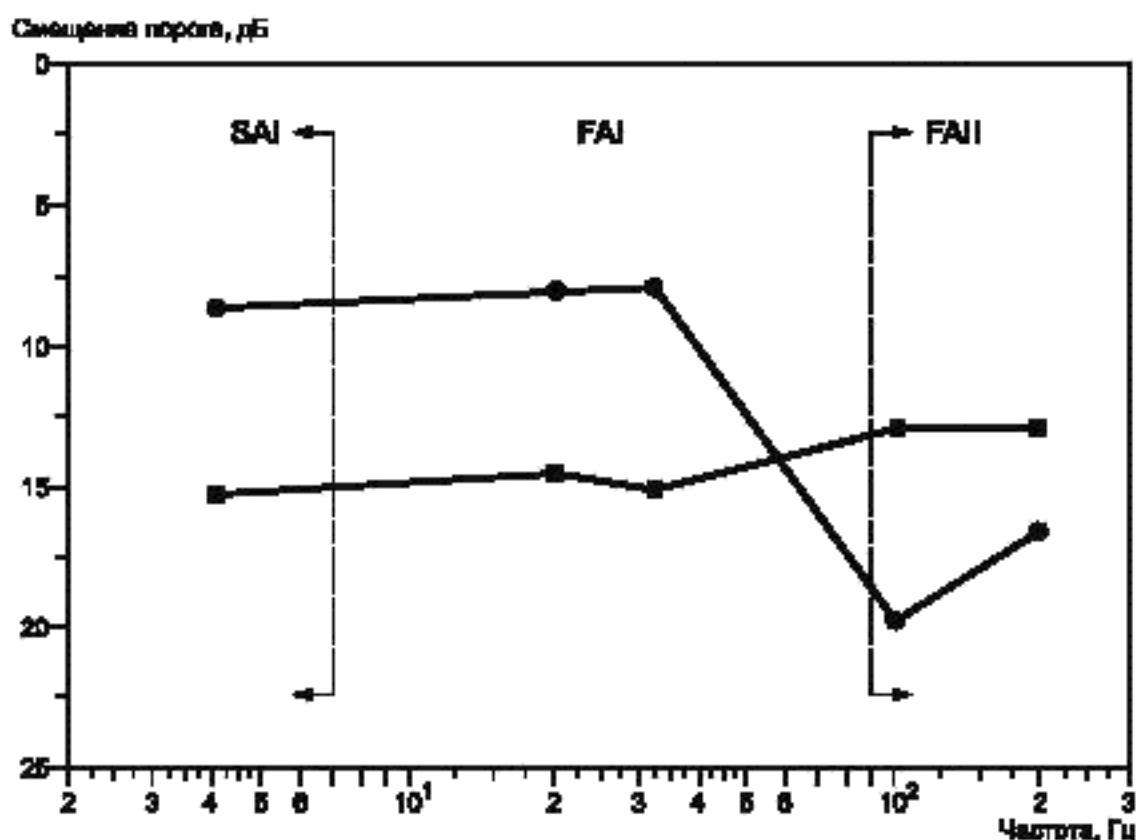
Рисунок В.1 — Тактограммы референтного смещения порога на пальцах двух операторов цепных лил
