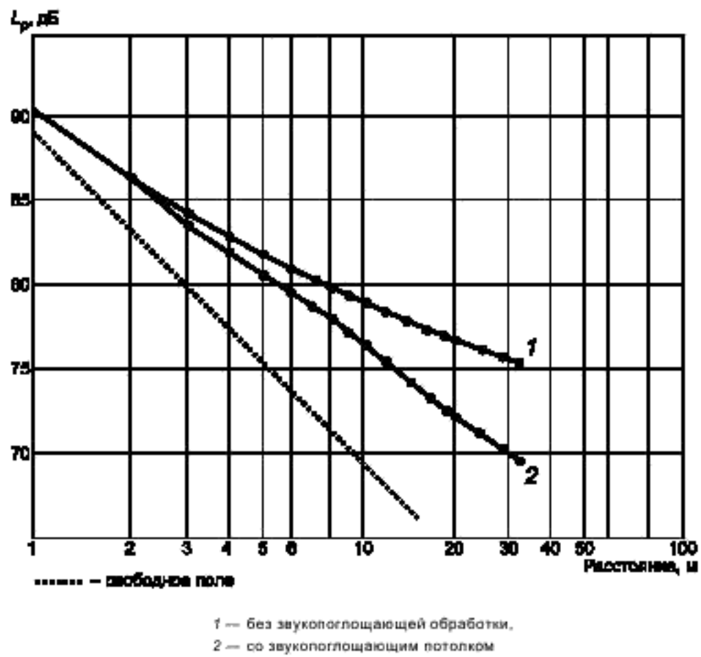
Рисунок D.1 — Рассчитанные линии пространственного распределения звука
