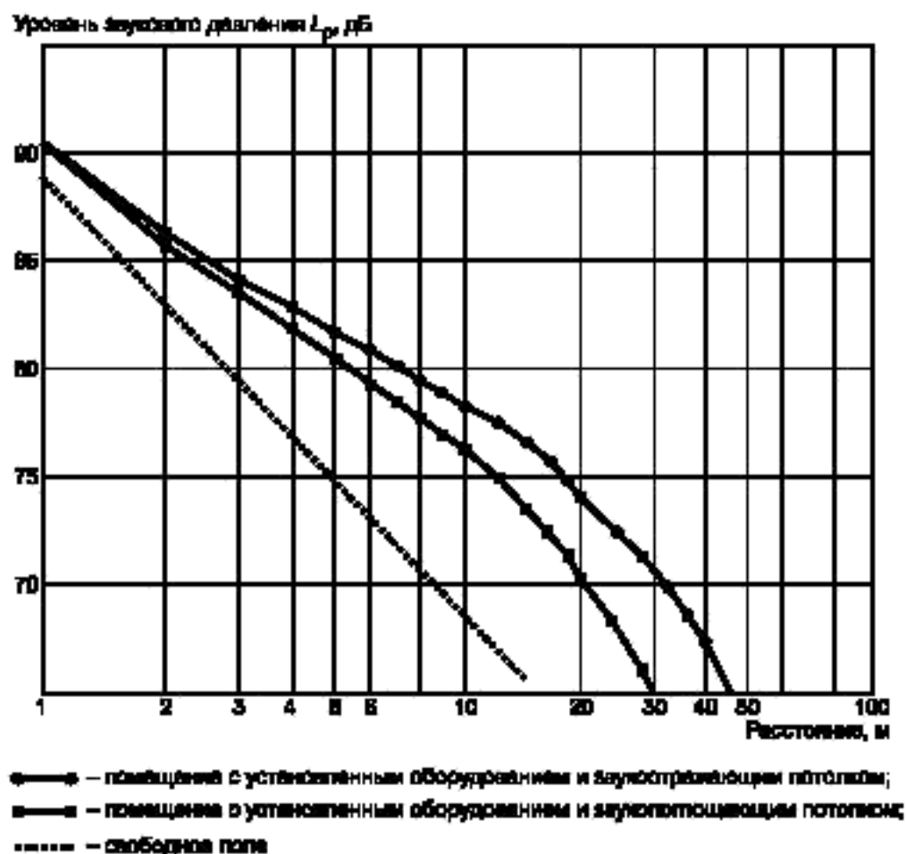
Рисунок 2 — Типичные линии пространственного распределения звука, излученного ненаправленным точечным источником звуковой мощностью 100 дБ в плоском заполненном оборудованием помещении со звукопоглощающим и со звукоотражающим потолком
