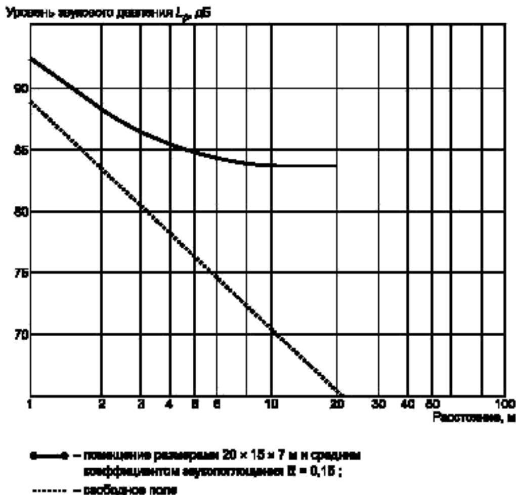
Рисунок В.2 — Расчетная линия пространственного распределения звука. Уровень звуковой мощности источника равен 100 дБ
