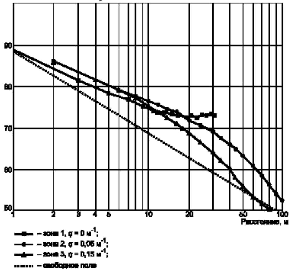
Уровень звукового давления L_p , дБ
