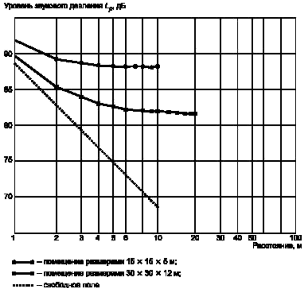
Рисунок 1 — Примеры линий пространственного распределения звука для двух помещений, имеющих различные размеры и одинаковые коэффициенты звукопоглощения
