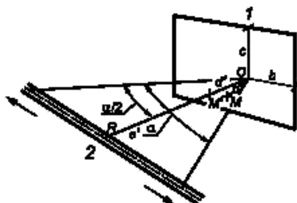
1 — фасад здания или другая звукоотражающая поверхность; 2 — протяженный источник шума; d — расстояние по перпендикуляру, опущенному из точки расположения микрофона на звукоотражающую поверхность; RO — биссектриса угла \alpha
