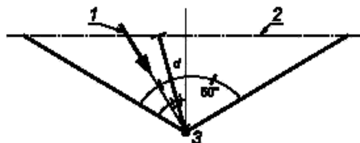
1 — среднее направление ветра; 2 — осевая линия дороги; 3 — микрофон
