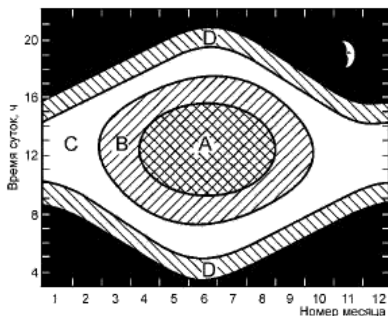
Рисунок А.3 — Временные интервалы, когда высота солнца в зависимости от месяца года и, следовательно, температурный градиент находятся в известных пределах (для 56^\circ северной широты. Для других широт — см. рисунок А.4)
