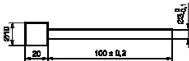
Рисунок 101 — Испытательный стержень для скрытой блокировки
