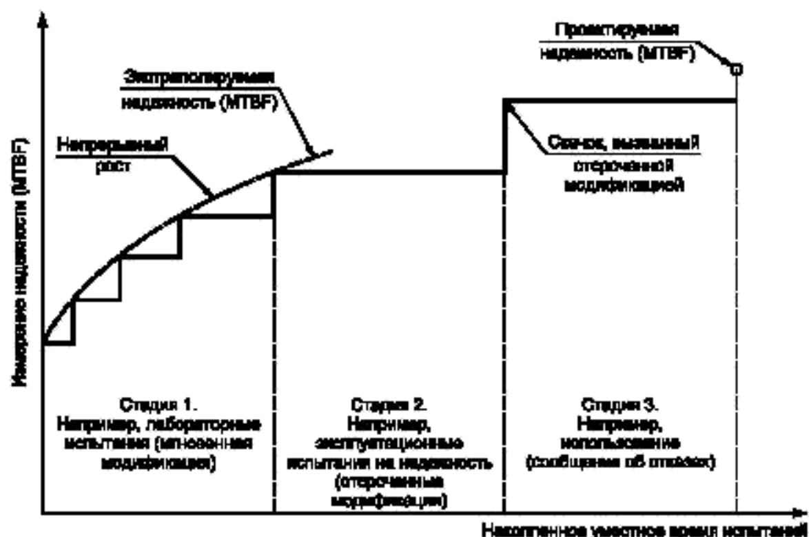
Рисунок 10 — Примеры кривых повышения надежности и скачков
