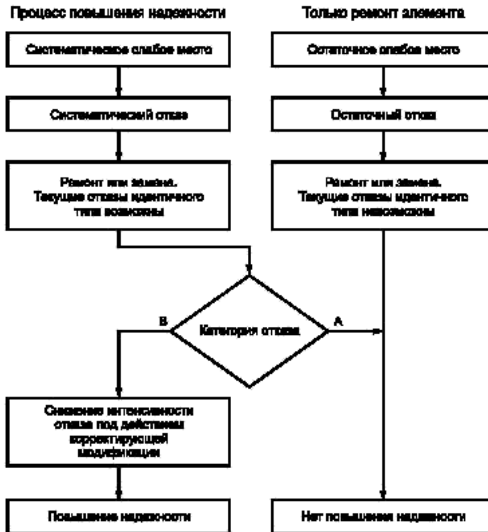
Рисунок 1 — Сравнение процесса повышения надежности и ремонта
