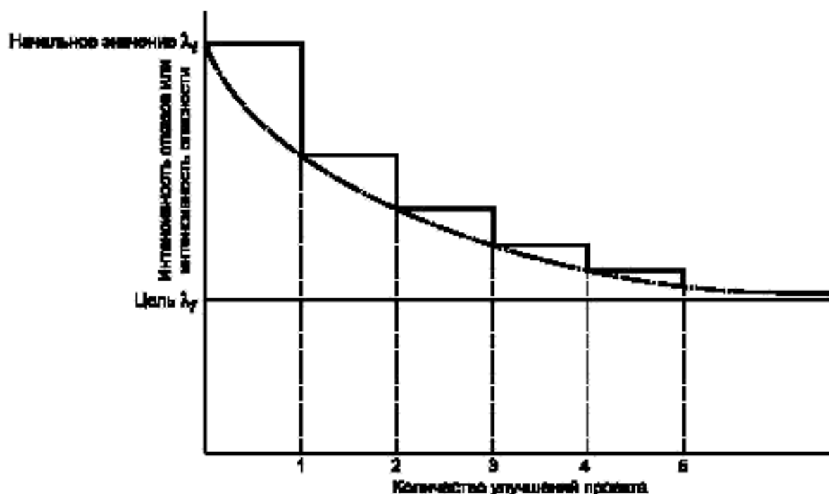
Рисунок 2 — Запланированное улучшение (снижение) эквивалентной интенсивности отказов
