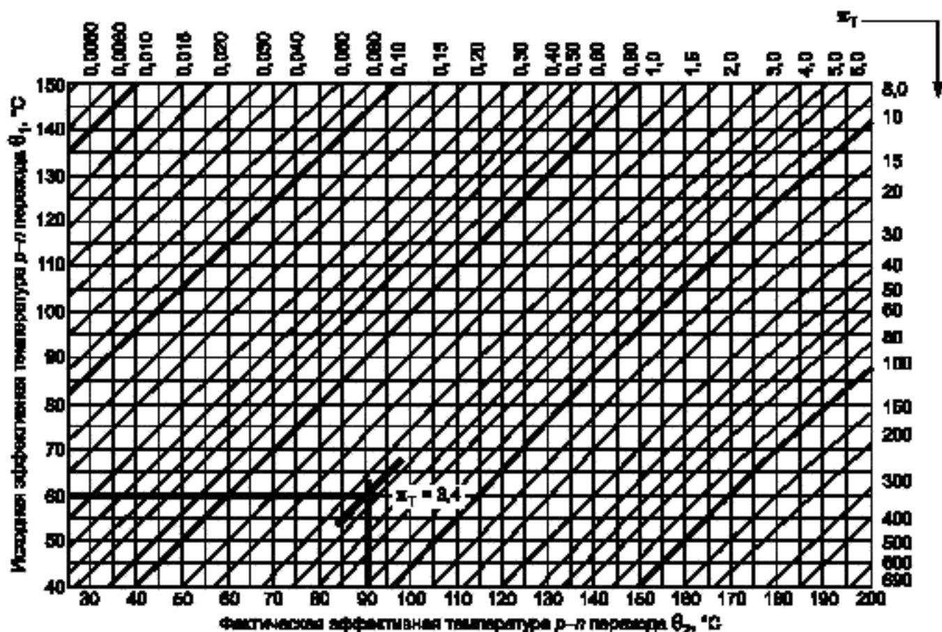
Рисунок А.1 — Зависимость интенсивности отказов от температуры
