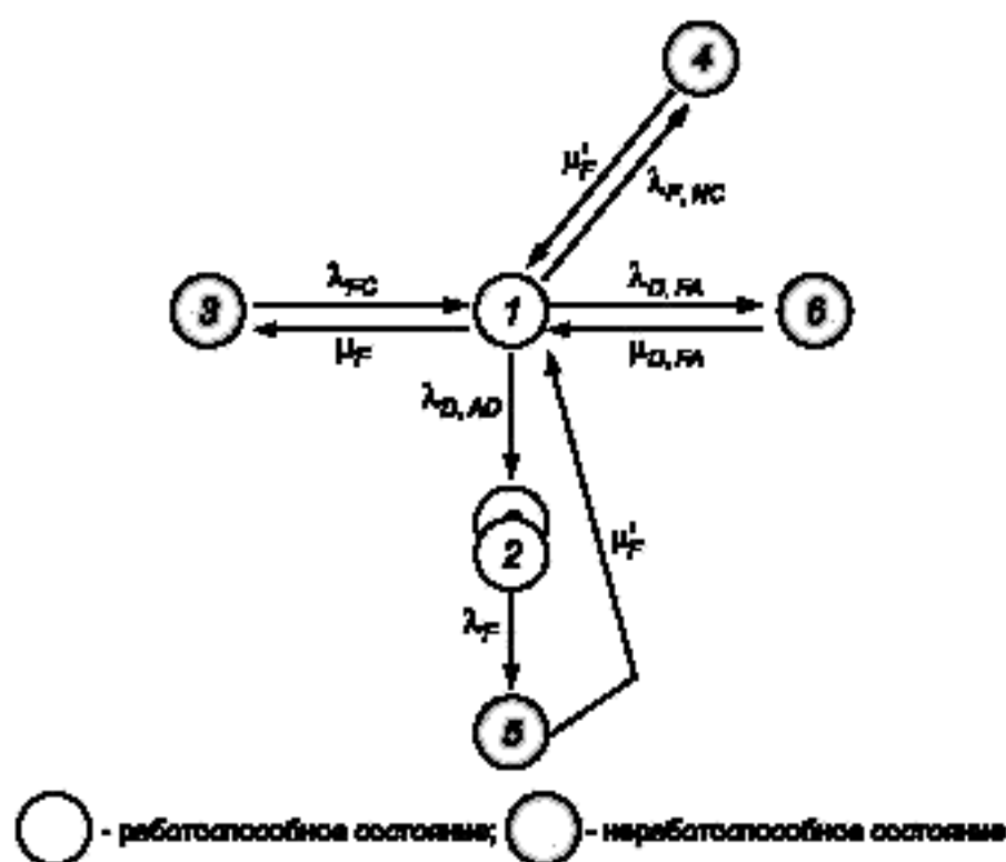
Рисунок А.7 — Диаграмма состояний и переходов
