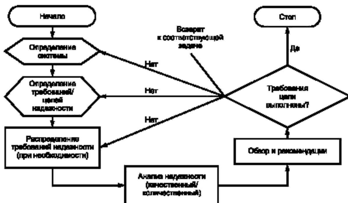
Рисунок 1 — Общая процедура анализа надежности
