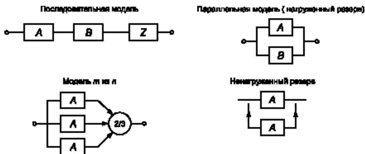
Рисунок A.5 — RBD для независимых блоков
