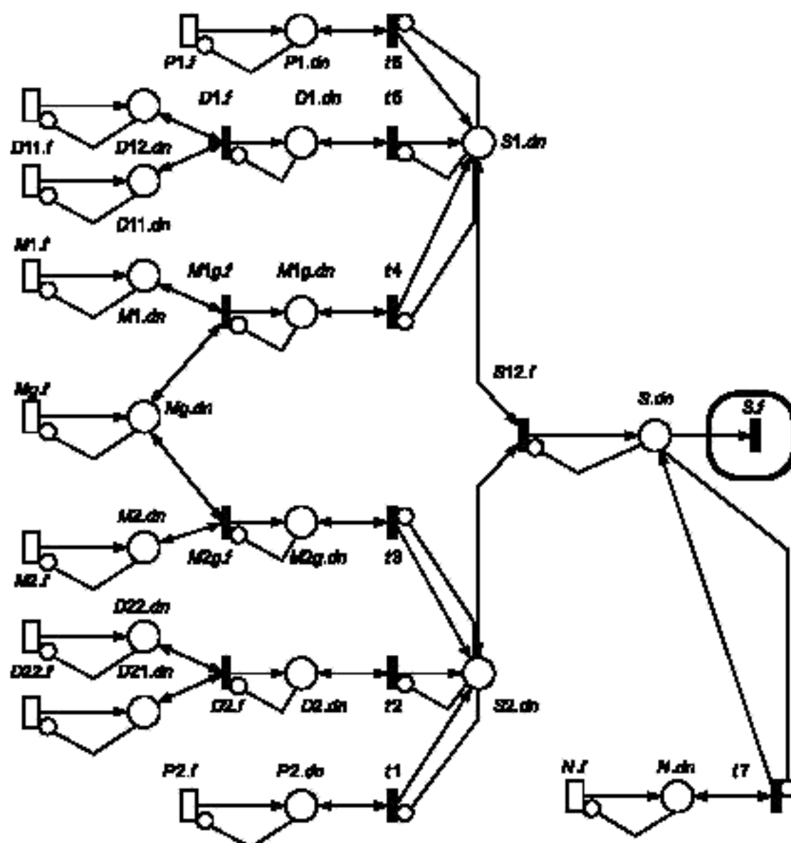
Рисунок А.9 — Сеть Петри мультипроцессорной системы
