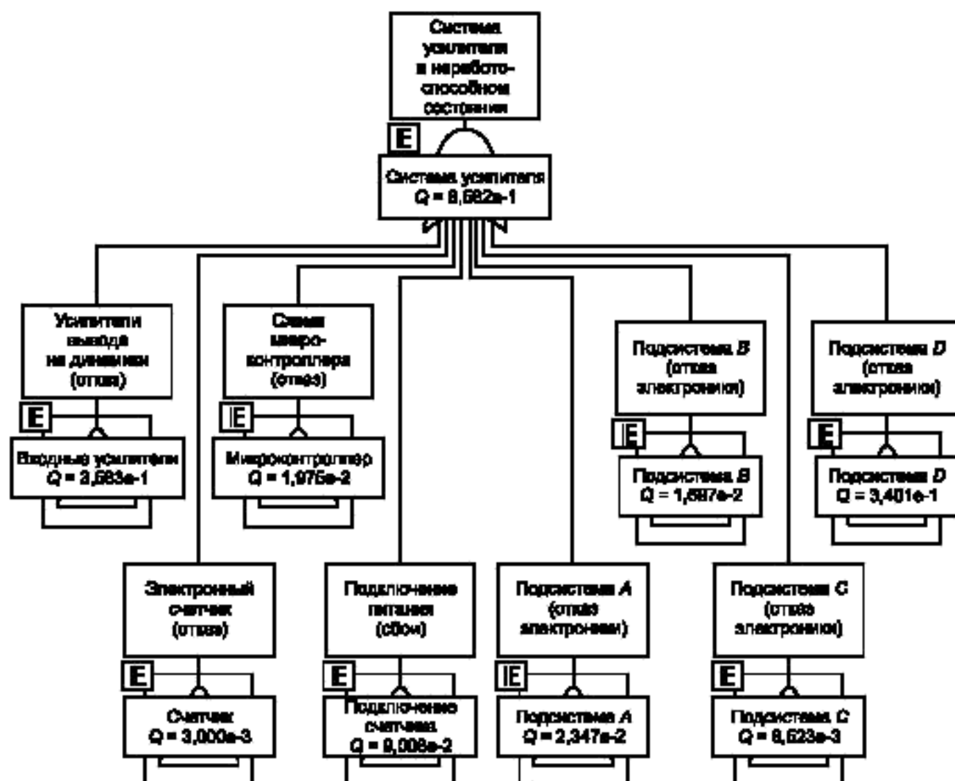
Рисунок А.2 — Дерево неисправностей для аудиоусилителя
