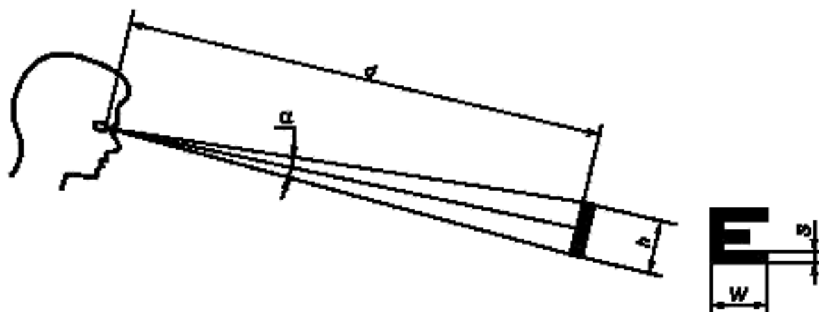
d – расстояние между глазом и знаком; \alpha – угол зрения знака . . . ; h – высота знака; w – ширина знака; z – толщина линий знака
