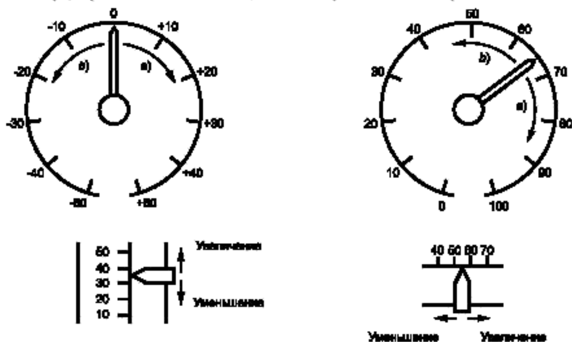
Рисунок 4 — Направления движения стрелок
