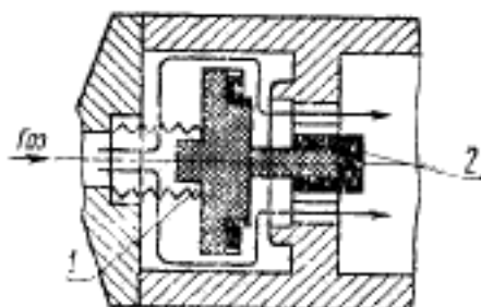
1 — пружина сжатия; 2 — плавкий элемент (например расплавляющийся припой)
