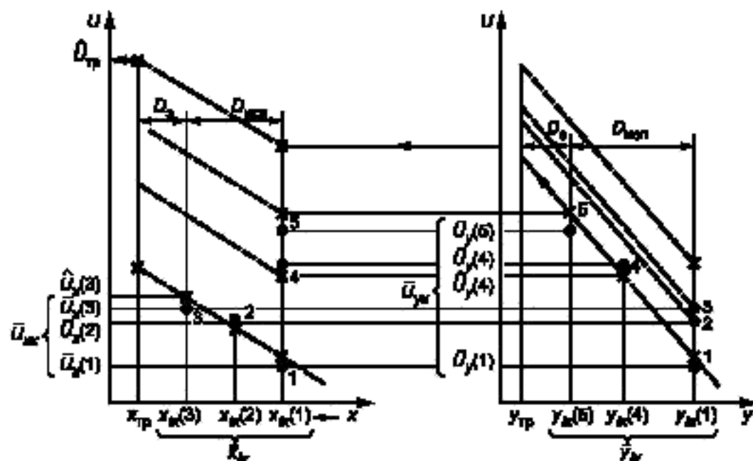
Рисунок А.1 — Схема эксперимента по варианту 1
