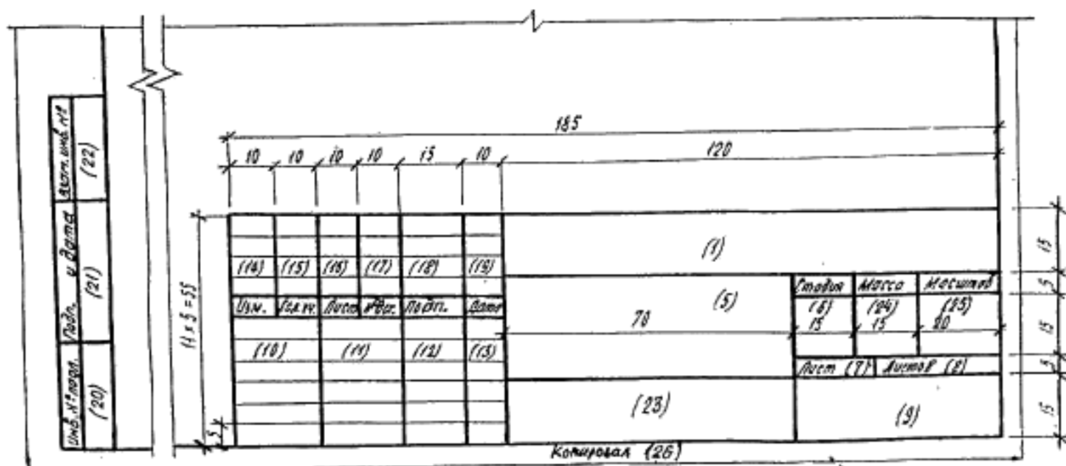
Форма 4 - Основная надпись и дополнительные графы к ней для чертежей строительных изделий (первый лист)
