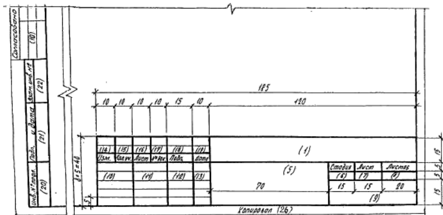
Форма 5 - Основная надпись и дополнительные графы к ней для всех видов текстовых документов (первые листы)
