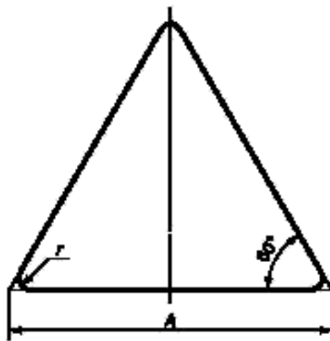
Рисунок Д.1 — Размеры треугольных знаков
