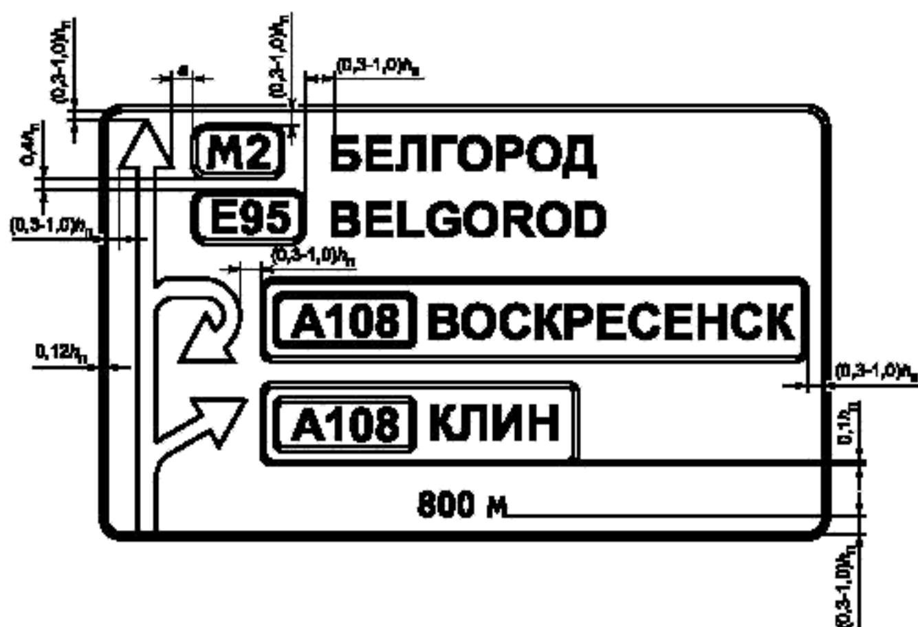
Рисунок Г.3 — Пример компоновки знака индивидуального проектирования 6.9.1
