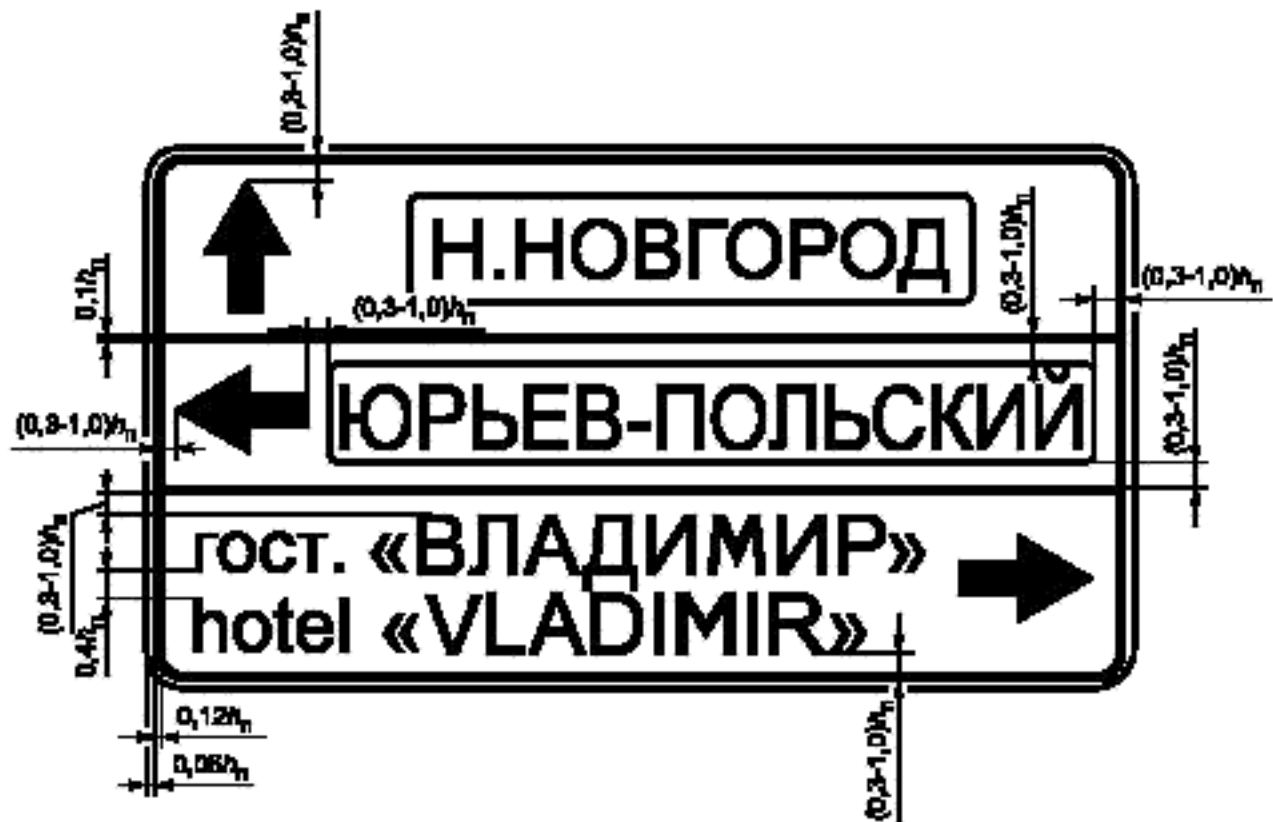
Рисунок Г.4 — Пример компоновки знака индивидуального проектирования 6.10.1
