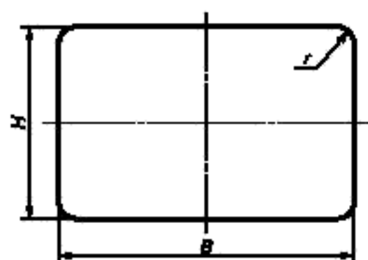
Рисунок Д.8 — Размеры прямоугольных знаков горизонтального формата
