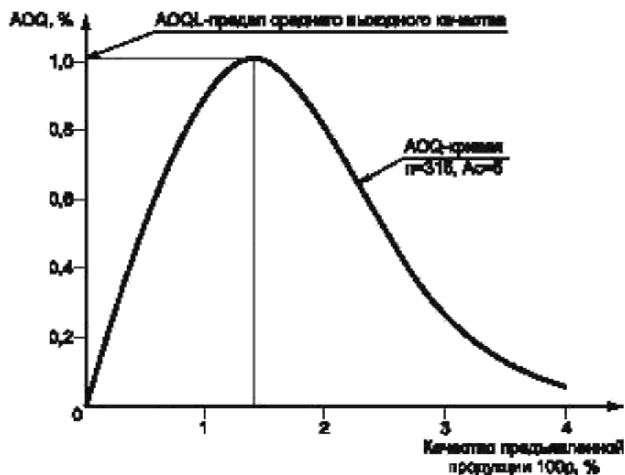
Рисунок 1 — AOQ и его предел AOQL
