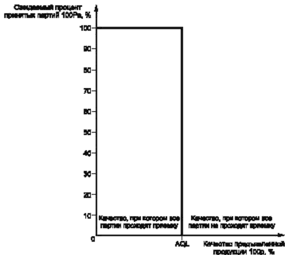
Рисунок 7 — Идеальная кривая оперативной характеристики
