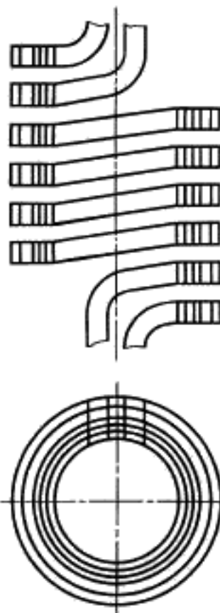
Двухходовая винтовая обмотка трансформатора (к термину 7.2.13)
