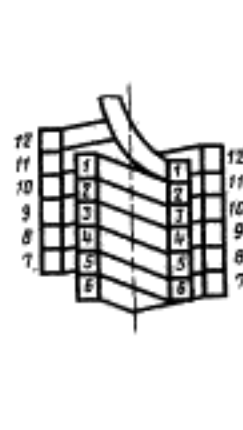
Двухслойная цилиндрическая обмотка трансформатора (к термину 7.2.5)
