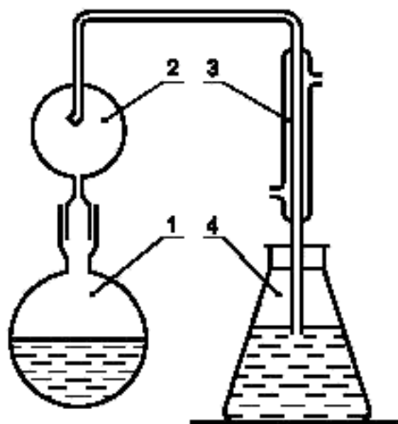
1 - круглая колба; 2 - каплеуловитель; 3 - холодильник; 4 - приемная колба
