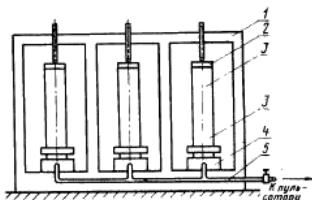
1—рама машины; 2—верхний винтовой овор с оголовником; 3—образец; 4—гидрозомкрат; 5—масляный провод.
