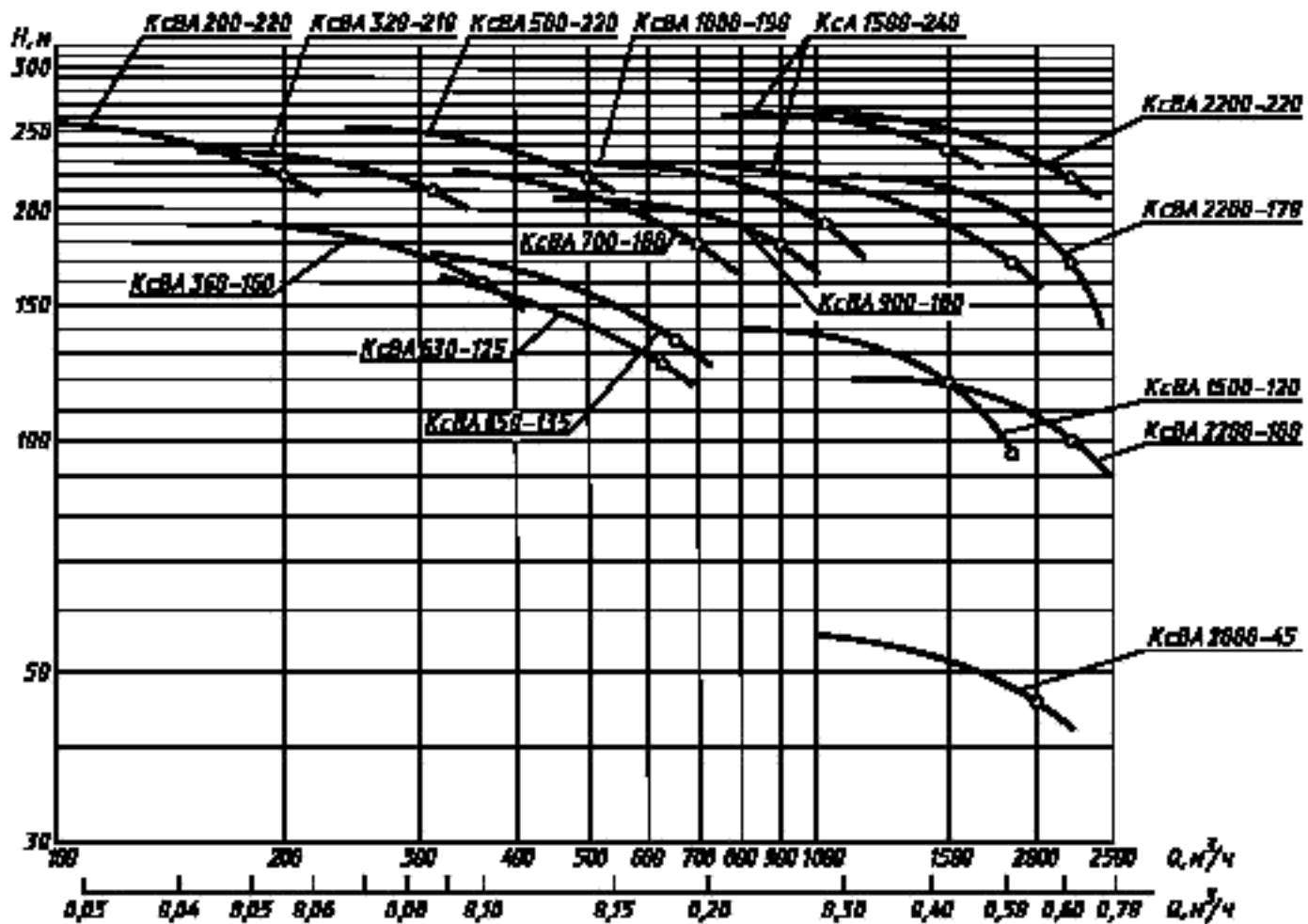
Рабочие части характеристик Q-H
