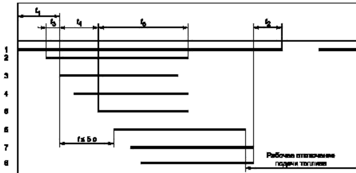
Диаграмма нормальной работы горелки
