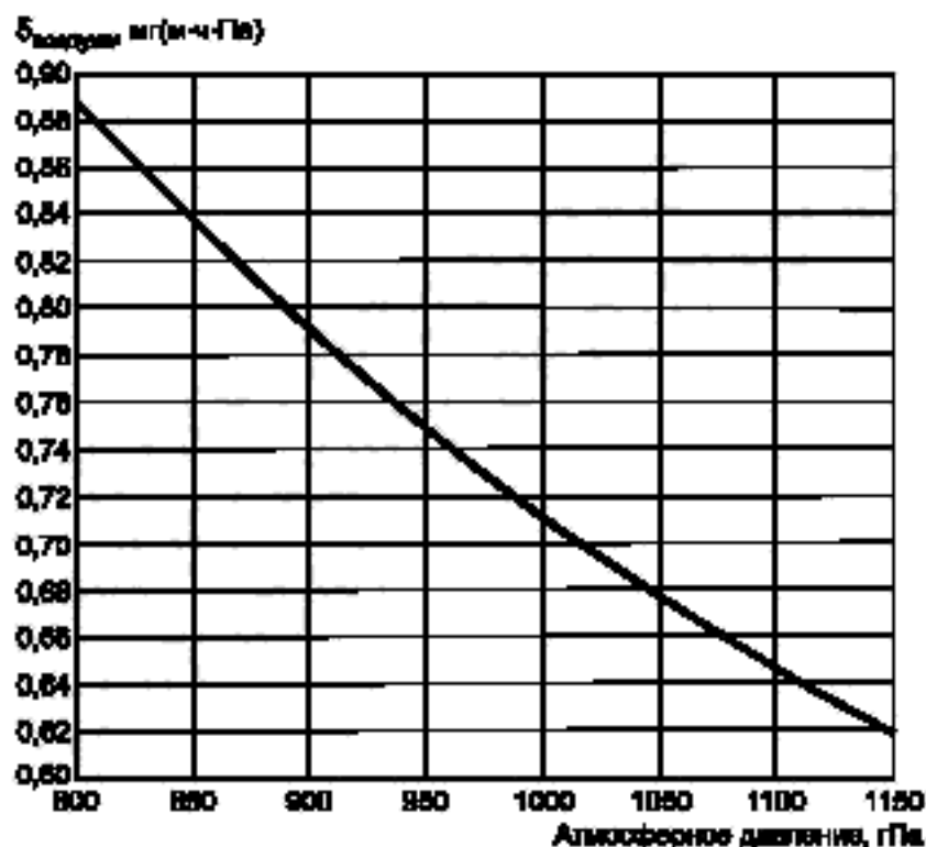
Рисунок 1 — Паропрооницаемость воздуха при 23 °C
