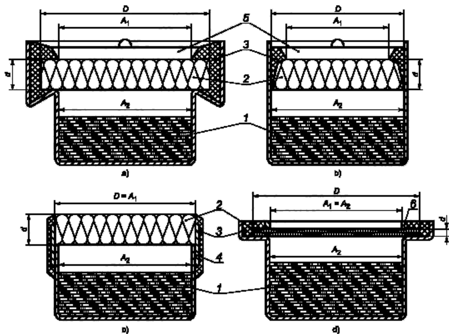
Типы испытательных чашек
