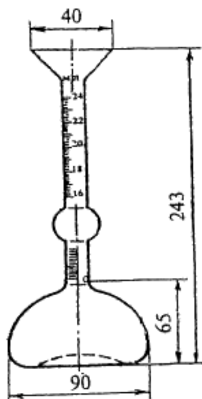
Рисунок 1 — Прибор Ле-Шателье
