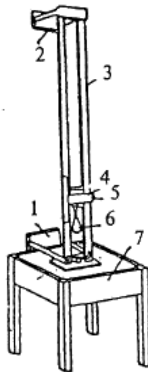
Рисунок 4 — Копер для испытания на ударное воздействие
