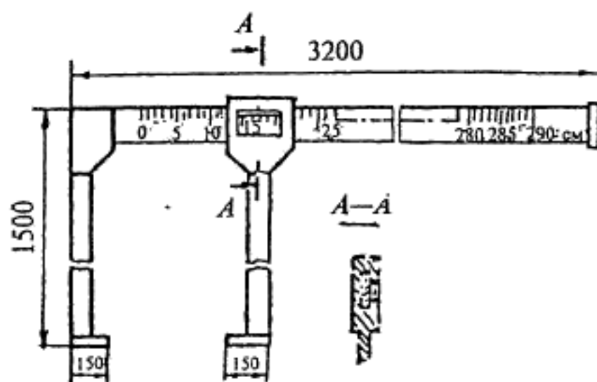
Рисунок 8 — Измерительный шаблон
