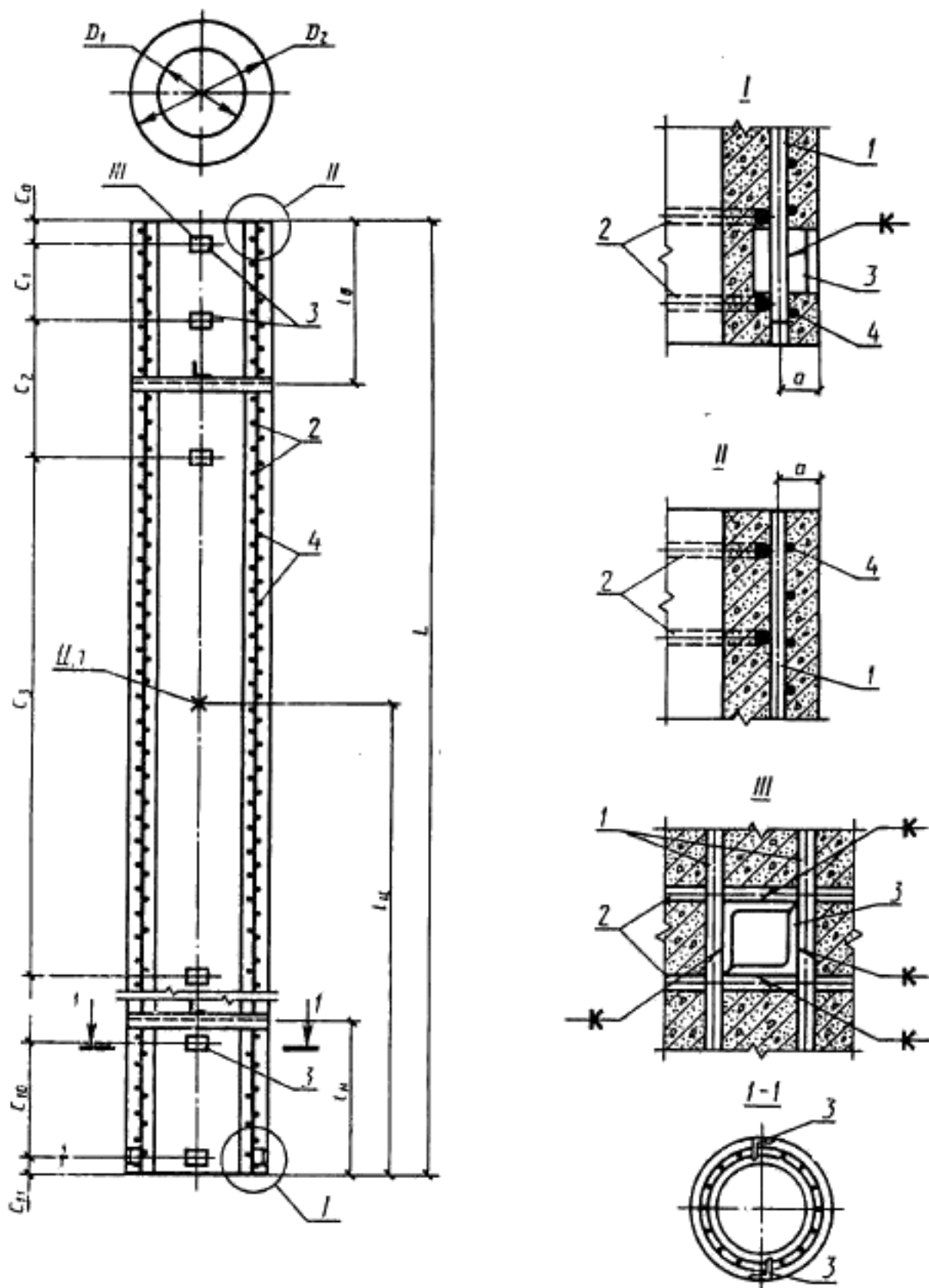
1 — продольная арматура; 2 — монтажные кольца; 3 — закладные изделия; 4 — спираль; a — расстояние от наружной поверхности стойки до оси продольной арматуры; c_0-c_1, c_{10}-c_{11} — привязка закладных изделий; ц. т. — центр тяжести; L — длина стойки; I_0 — расстояние до центра тяжести; I_1, I_2 — расстояния до мест установки диафрагмы; D_1 — внутренний диаметр стойки; D_2 — наружный диаметр стойки
