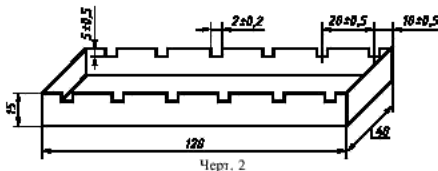
Подставка для старения образцов
