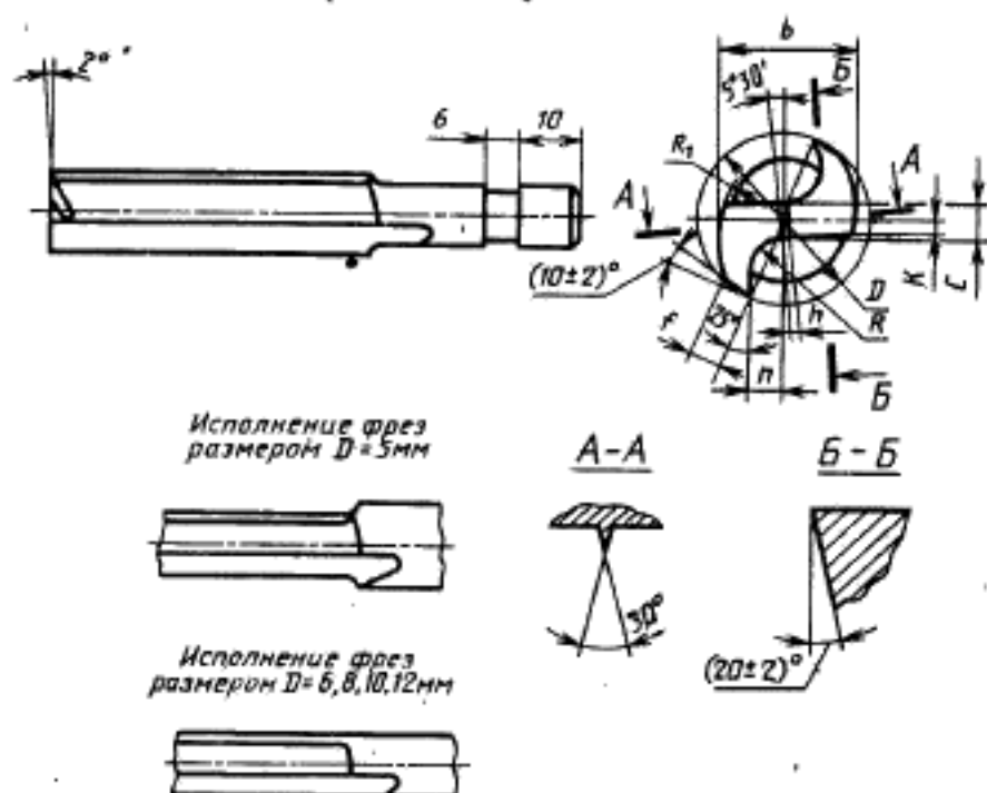
Фреза типа 2 с прямой канавкой
