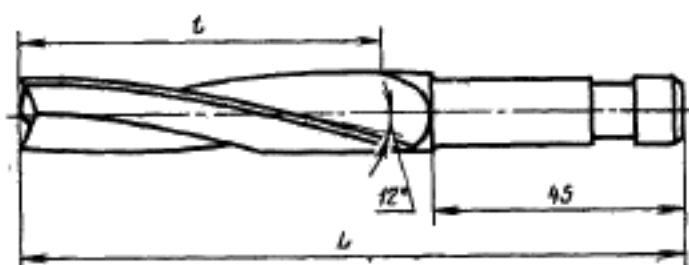
Размеры, мм
