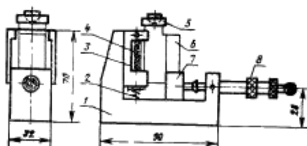
1—корпус; 2—пружина; 3—подвижная вилка; 4—ролики; 5—нажимная призма с шаровой опорой; 6—образец; 7—подвижная опора; 8—устройство для прижима подвижной опоры
