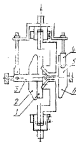
1 — образец; 2 — удерживающая планка; 3 — планка; 4 — захват; 5 — упор; 6 — траверса
