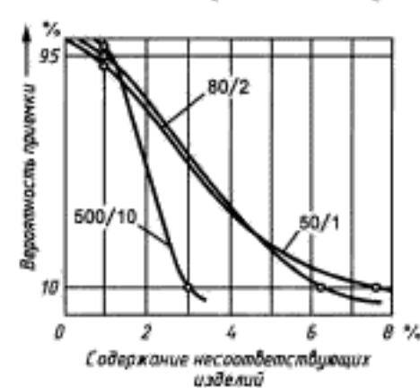
Кривые оперативных характеристик для планов выборочного контроля
