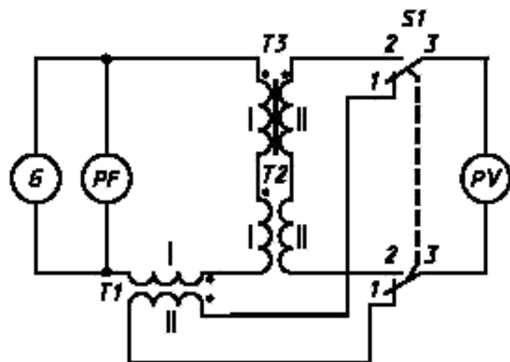
Рисунок 1 — Схема для измерений в динамическом режиме перемагничивания
