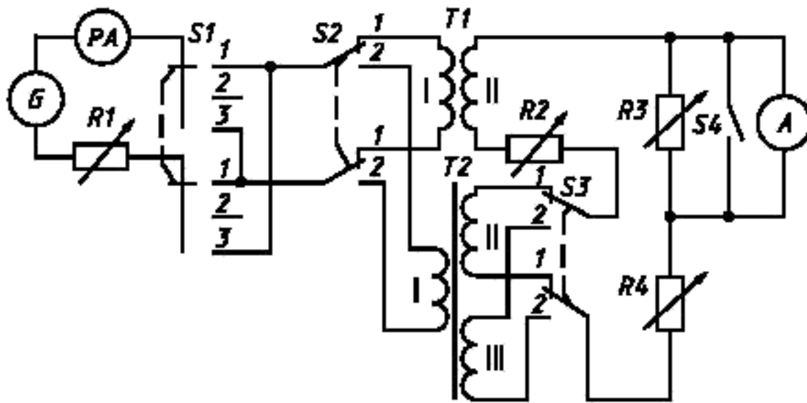
Рисунок 1 — Схема для измерений в пермеамetre
