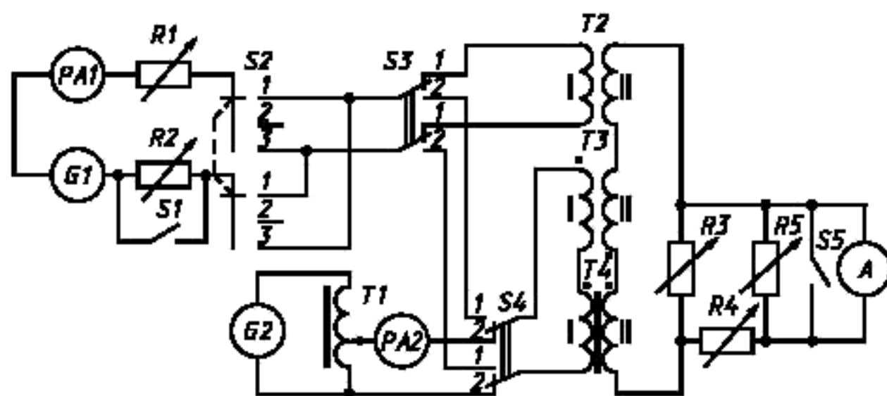
Рисунок 1 — Схема для измерений в постоянном магнитном поле
