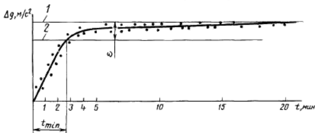
Определение длительности переходного процесса
