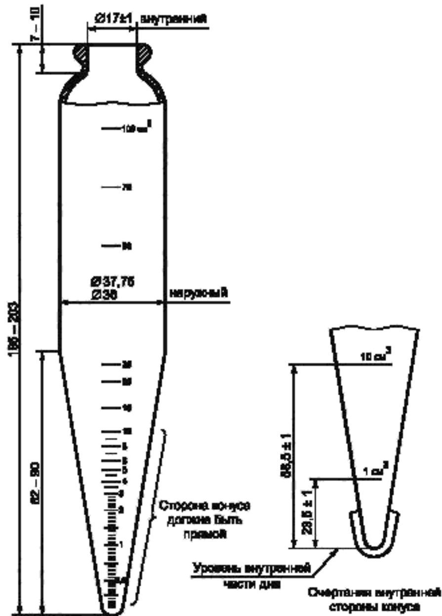
Рисунок 1 — Пробирка для центрифуги высотой 200 мм
