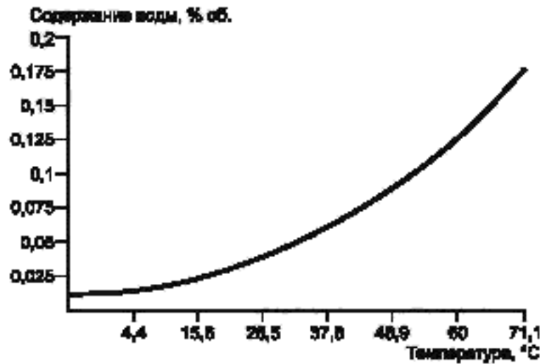
Рисунок В.1 — Растворимость толуола в воде
