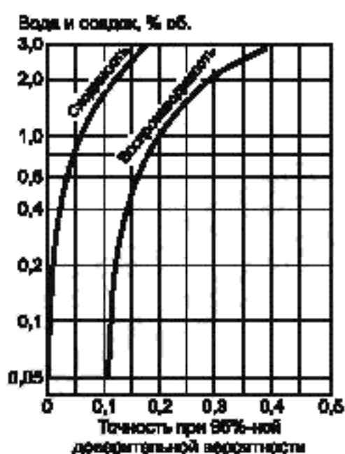
Рисунок 3 — Данные по прецизионности
