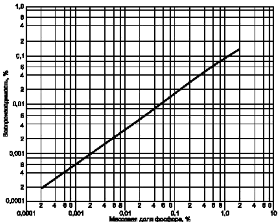
Рисунок 3 — Воспроизводимость фотометрического метода
