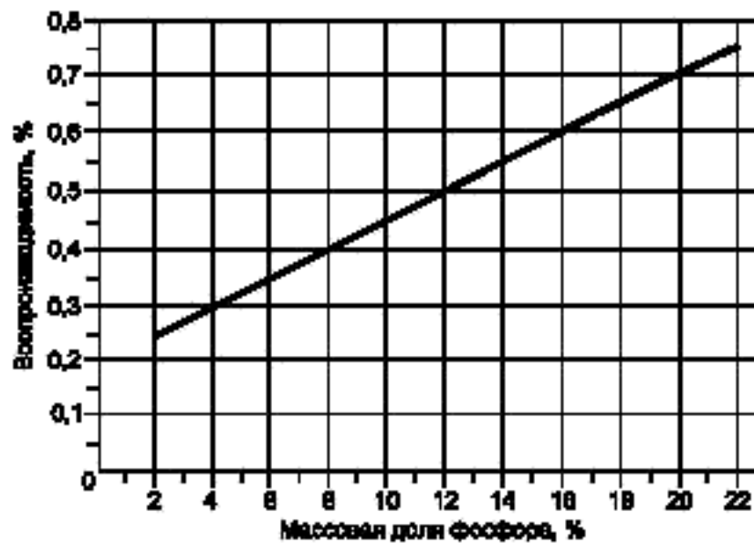
Рисунок 4 — Воспроизводимость гравиметрического метода
