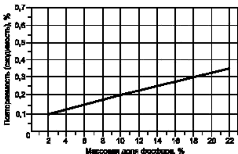
Рисунок 2 — Повторяемость (сходимость) гравиметрического метода
