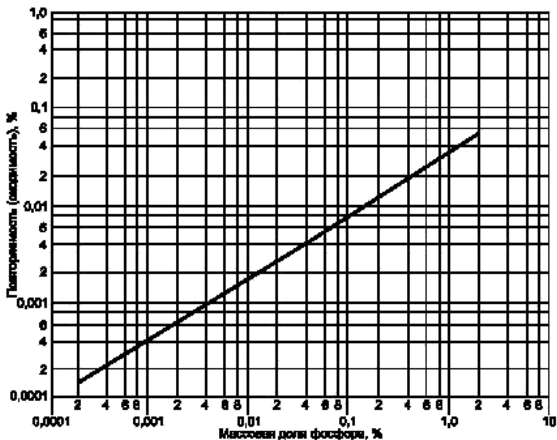
Рисунок 1 — Повторяемость (сходимость) фотометрического метода
