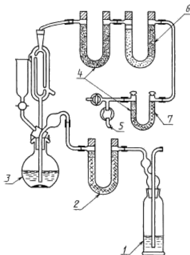
Установка для определения диоксида углерода
