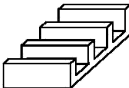
Рисунок 2 — Схема подставки для размещения образцов
