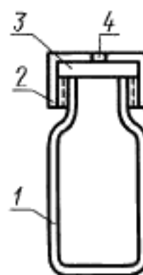
1 — сосуд; 2 — крышка; 3 — резиновая мембрана; 4 — отверстие в крышке
