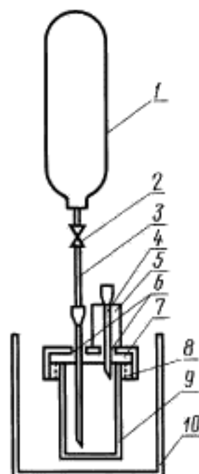
Схема подготовки сжиженного моноэтиламина
