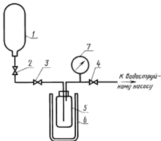
Схема подготовки сжиженного моноэтиламина
