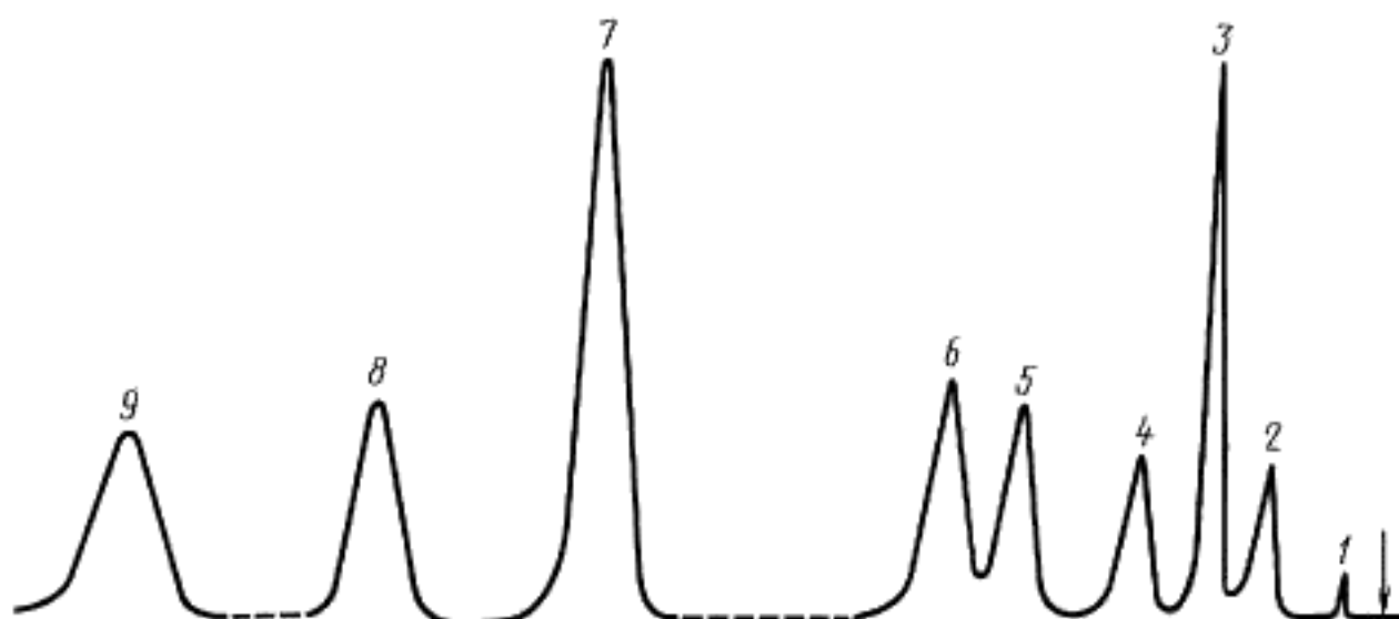
Хроматограмма искусственной смеси этиламинов
