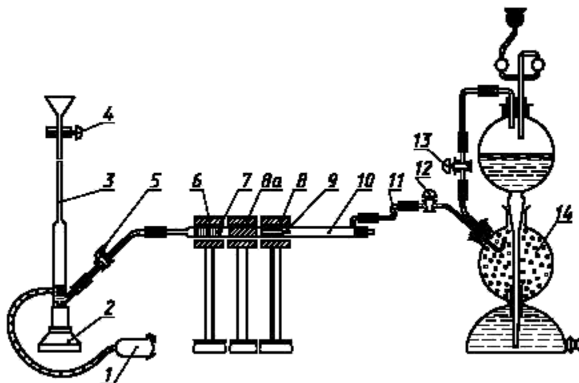
Схема установки для газометрического микроотделения азота
