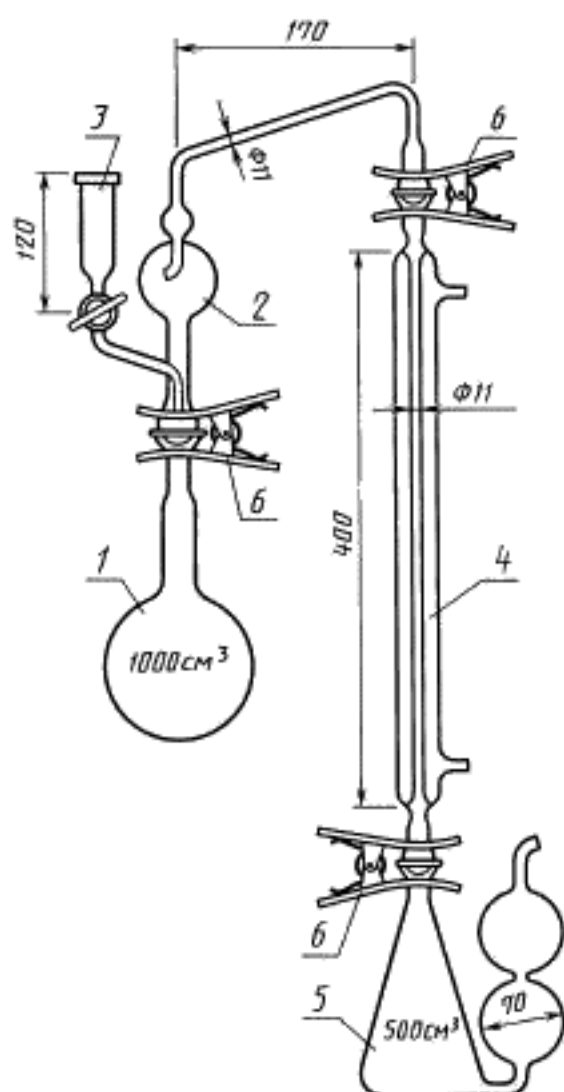
Дистилляционный аппарат
