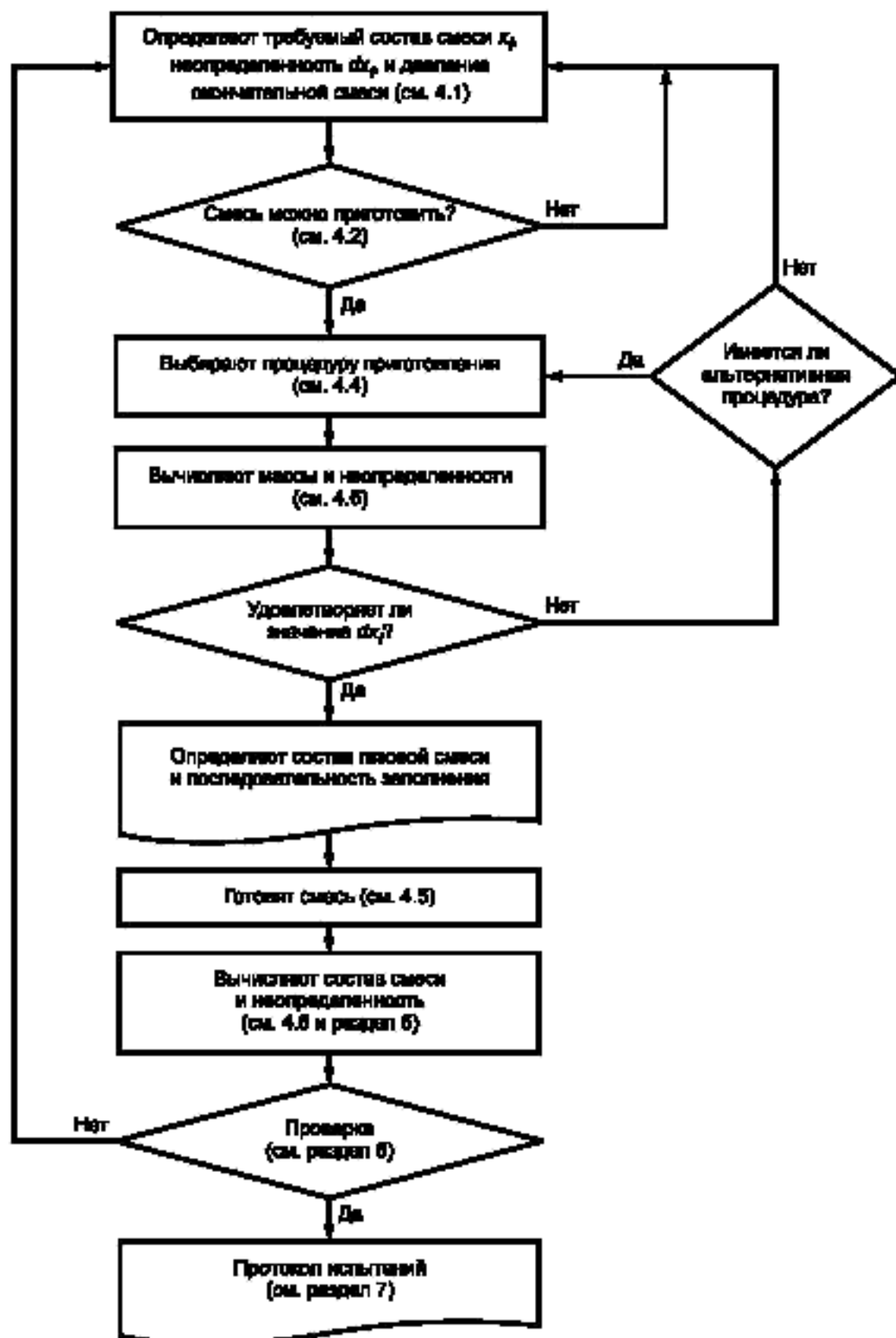
Рисунок 1 — Схема гравиметрического метода приготовления градуировочных газовых смесей
