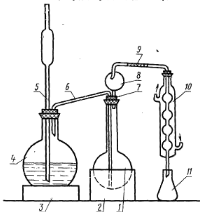
Прибор для перегонки водяным паром
