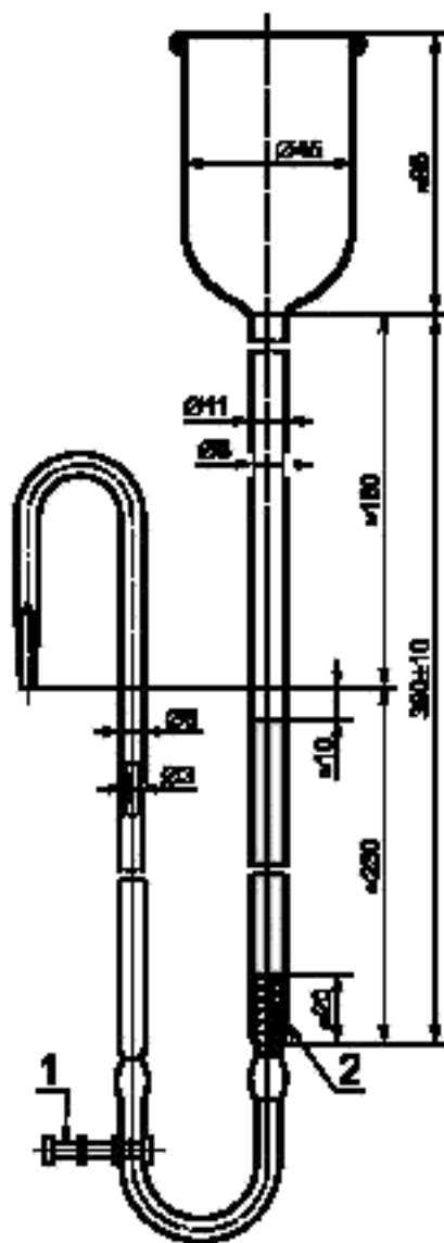
1 — зажим с винтом; 2 — прокладка из стекловаты
