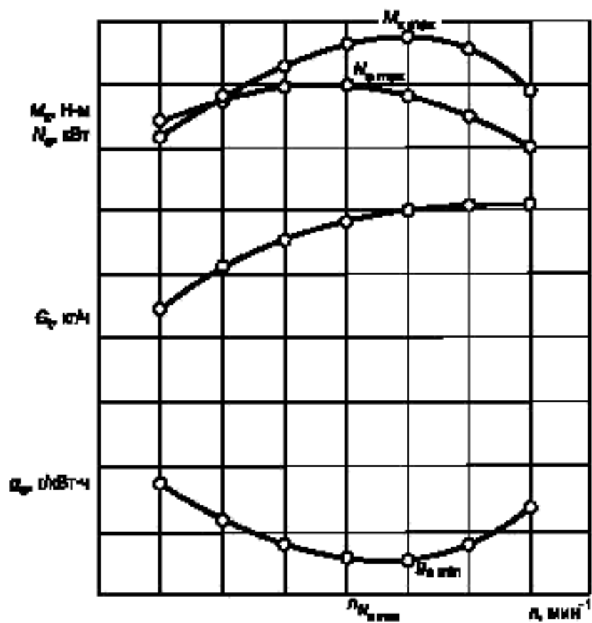
Рисунок Б.1 — Внешняя скоростная характеристика двигателя бензоинструмента
