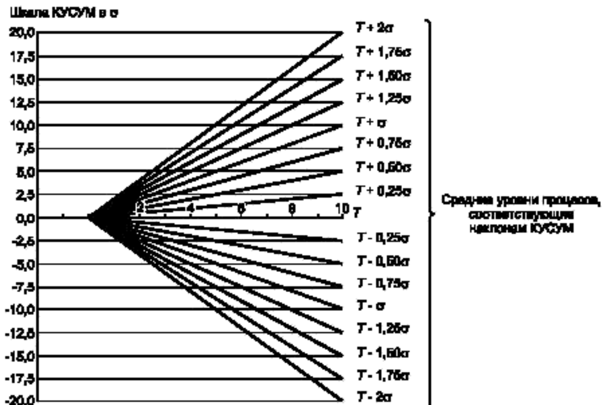
Рисунок Б.1 — Построение транспортира КУСУМ (указателя наклона) (для ясности показана нетипично крупная шкала)
