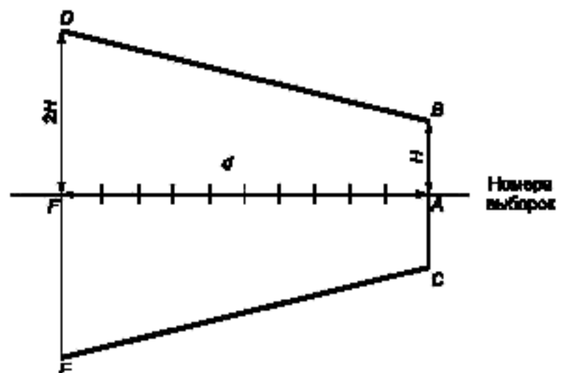
Рисунок 1 — Шаблон усеченной V-маски
