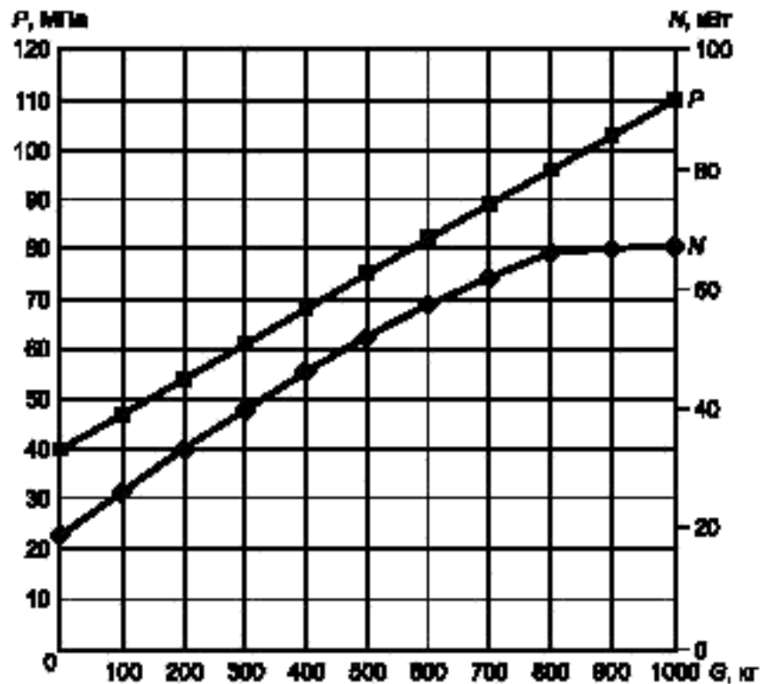
Рисунок 1 — Графическое изображение нагрузочной характеристики гидросистемы
