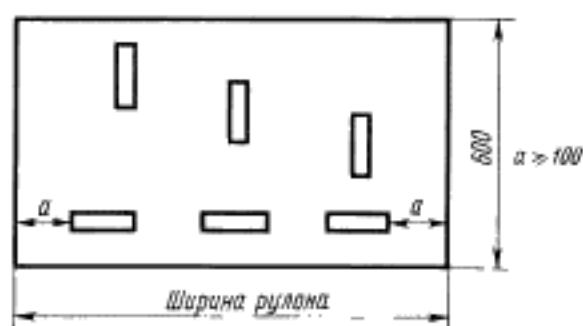
Схема раскроя
