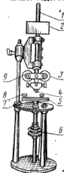
ПРИБОР ФЕДОРОВА
