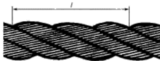
l — один шаг крутки 3-рядного каната
