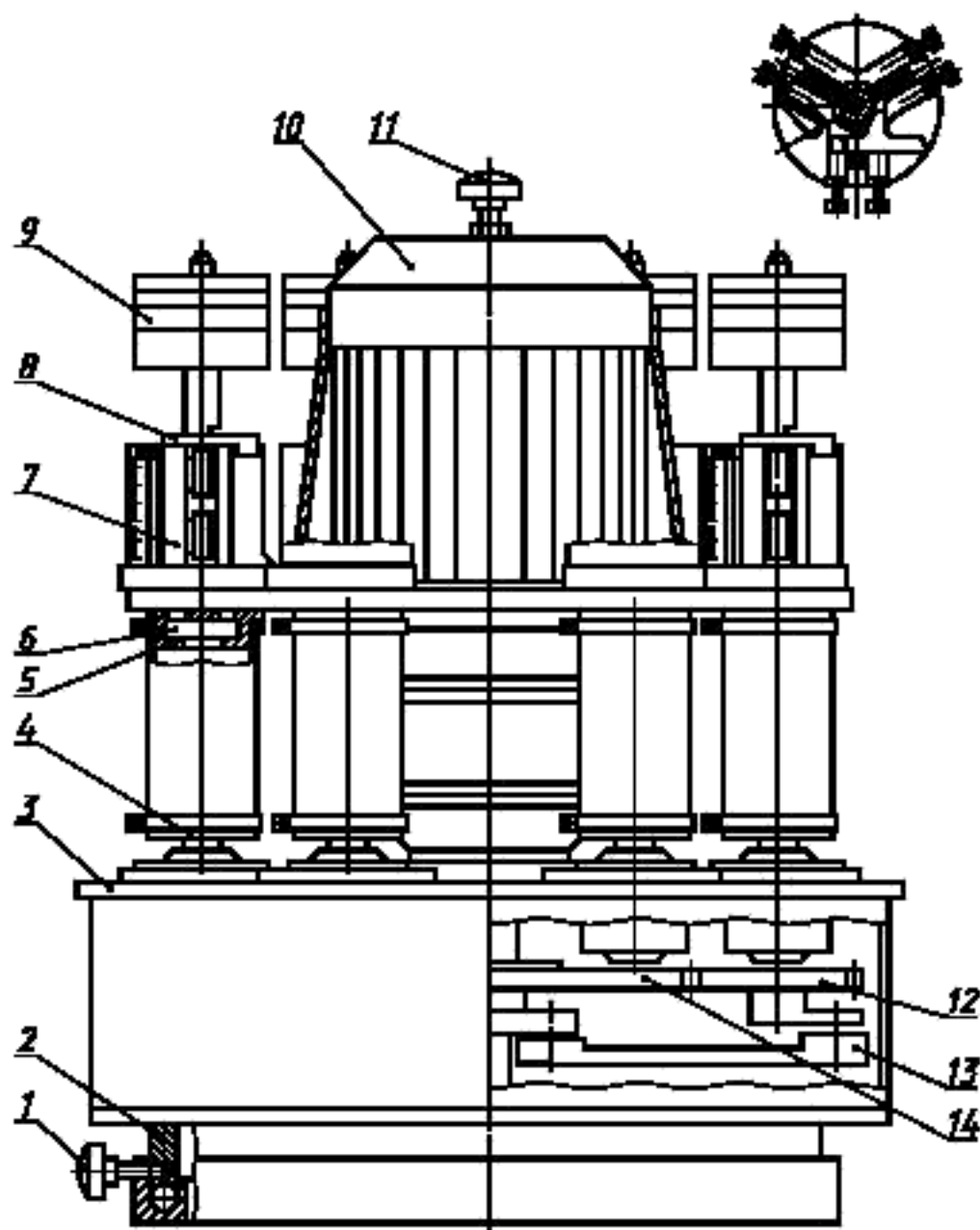
1 — стопорный винт; 2 — опора на шариках; 3 — основание; 4 — нижний зажим; 5 — верхний зажим; 6 — комут; 7 — направляющий корпус с подшипником; 8 — фиксатор; 9 — съемный груз; 10 — мотор-редуктор; 11 — маховичок; 12 — шестерня; 13 — шатун; 14 — шестерня
