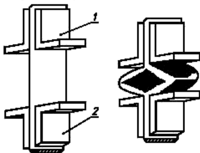
1 — неподвижный зажим; 2 — подвижный зажим
