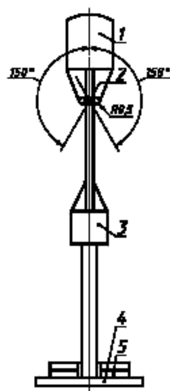
1 — верхний подвижный зажим; 2 — губки подвижного зажима; 3 — нижний подвижный зажим; 4 — площадка для грузов; 5 — грузы
