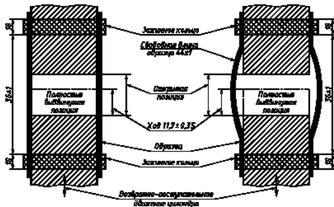
а) Стандартный образец 105 × 50 мм
