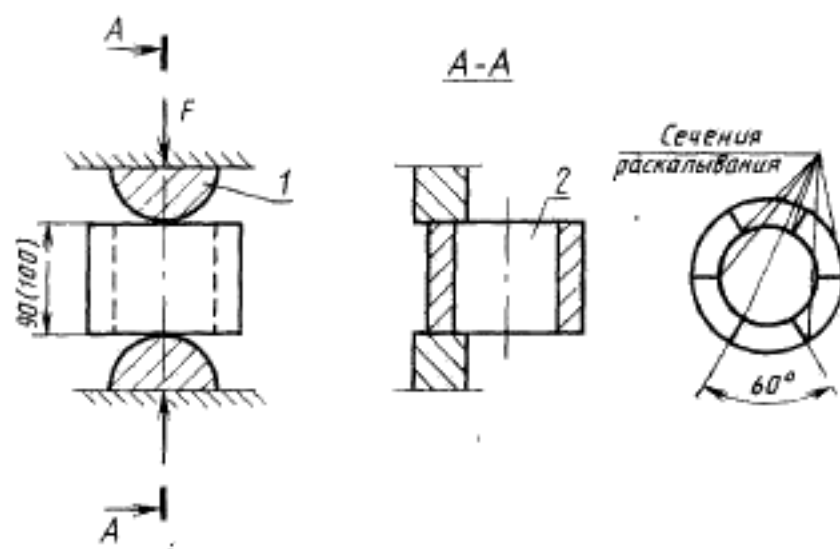
1—колющий полуцилиндр; 2—образец
