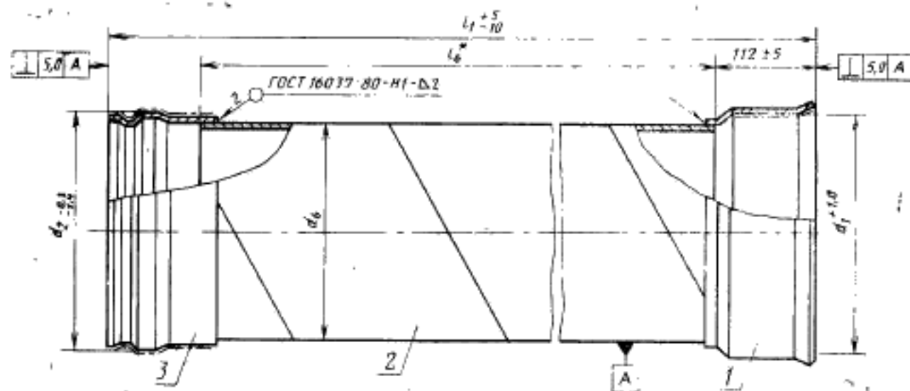
Сердечник трубы С25.50...С60.100
