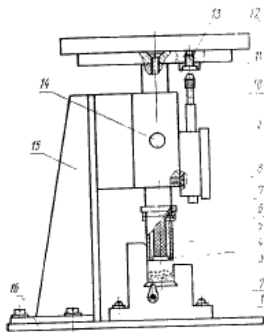
1—основание; 2—высоковольтный электрод; 3—проба нитей; 4—измерительный электрод; 5— изолятор; 6—охраняемый электрод; 7—пластина; 8—ось; 9—индикатор; 10—направляющая; 11—под- ставка; 12—груз; 13—винт; 14—фиксирующий винт; 15—кронштейн; 16—пластина
