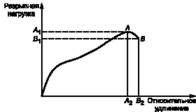
Рисунок 1 — Типичная кривая разрывная нагрузка — относительное удлинение
